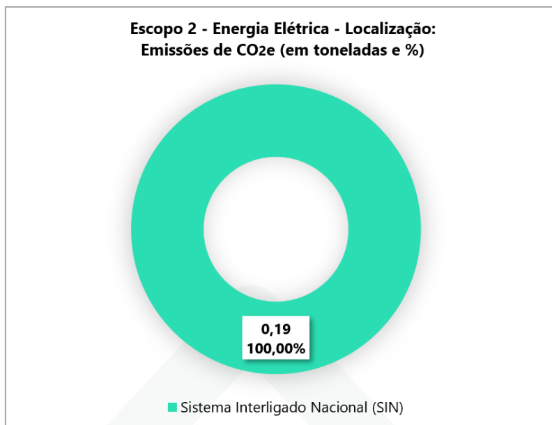
Gráfico 7 – Emissões de CO 2 e do Escopo 2 – Localização
