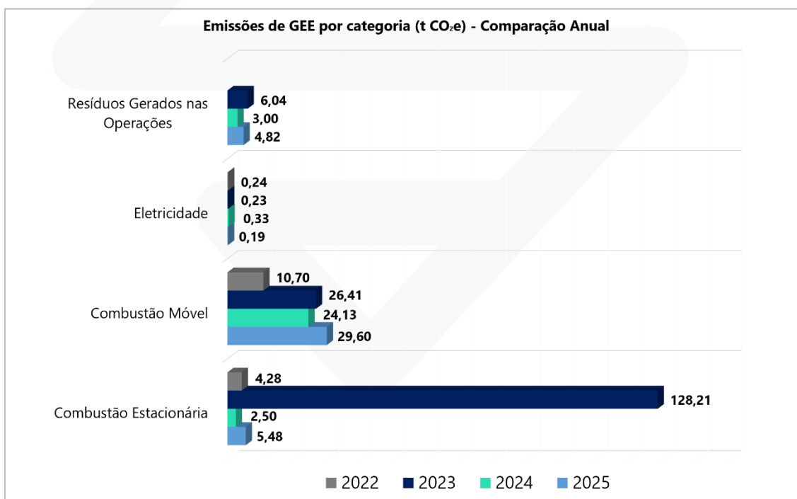
Gráfico 12 – Comparação do resultado de emissões de CO 2 e por Categoria entre os anos
