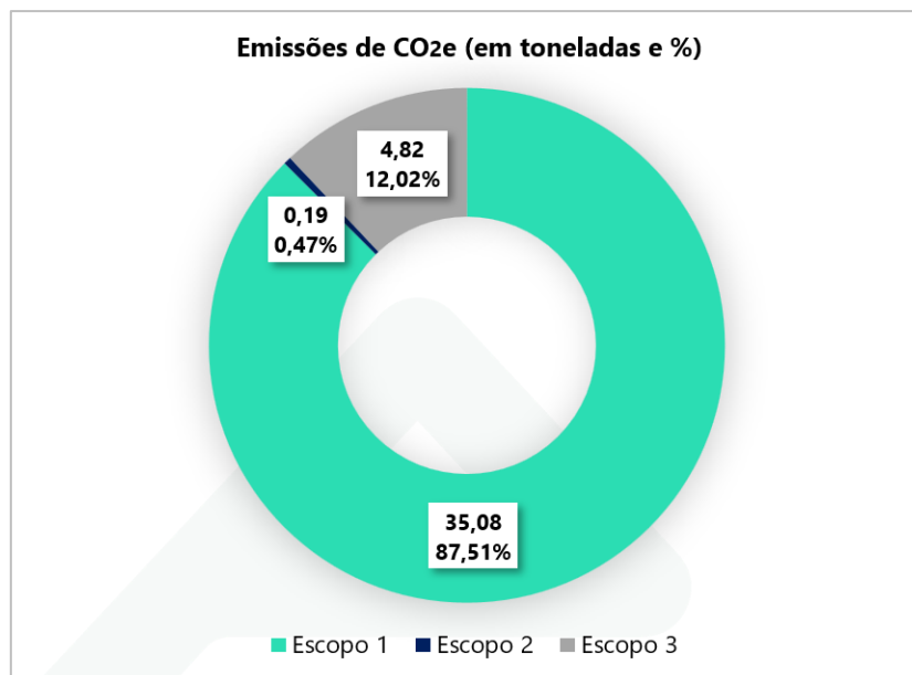
Gráfico 1 – Emissões de CO 2 e por escopo
