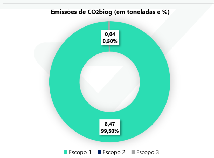
Gráfico 2 – Emissões de CO 2 biog por escopo
