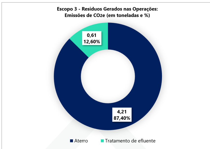
Gráfico 8 – Emissões de CO 2 e de Resíduos Gerados nas Operações (Escopo 3)
