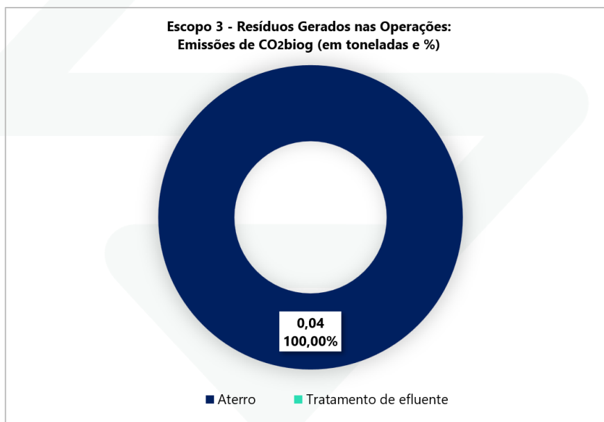
Gráfico 9 – Emissões de CO 2 biog de Resíduos Gerados nas Operações (Escopo 3)
